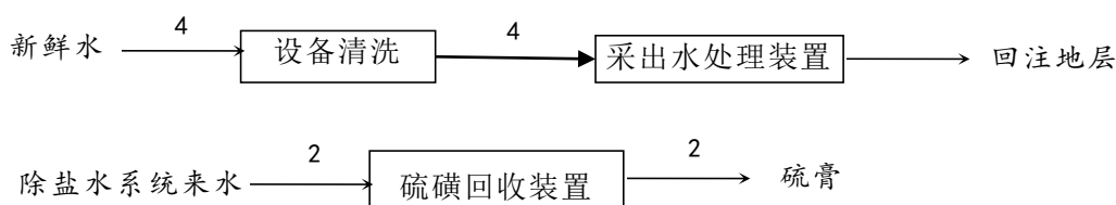
图3.2-1 拟建工程水平衡图 单位：m 3 /d
