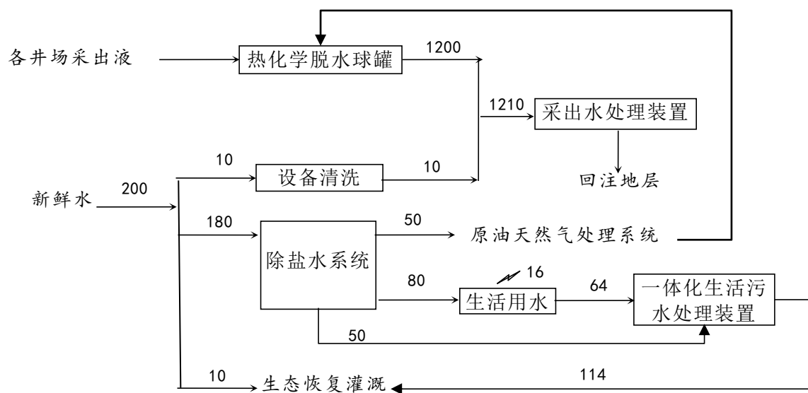
图 3.1-1 现有工程水平衡图 单位：m 3 /d
