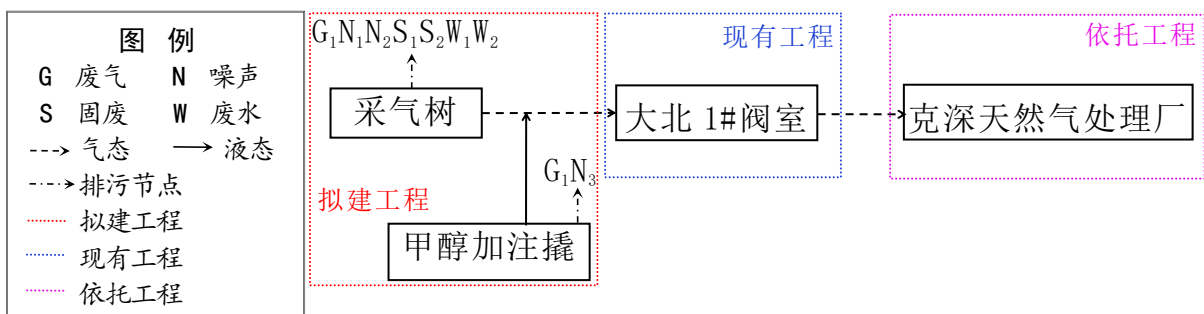
图 3.3-4 井场油气开采及集输工艺流程图
