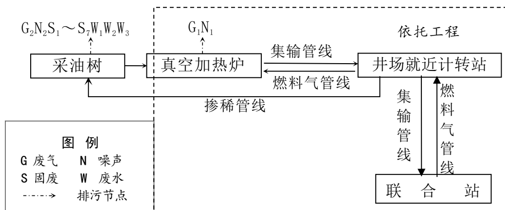
图 3.3-6 油气开采及集输工艺流程图
