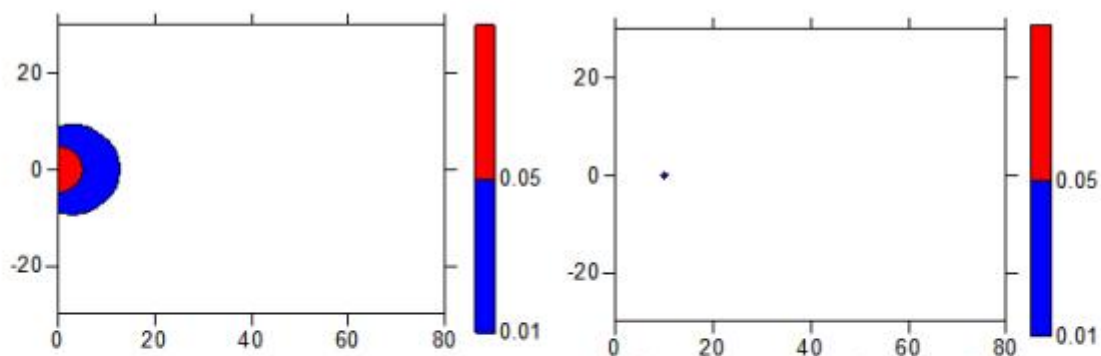
(1) 100d 时污染晕运移分布图
