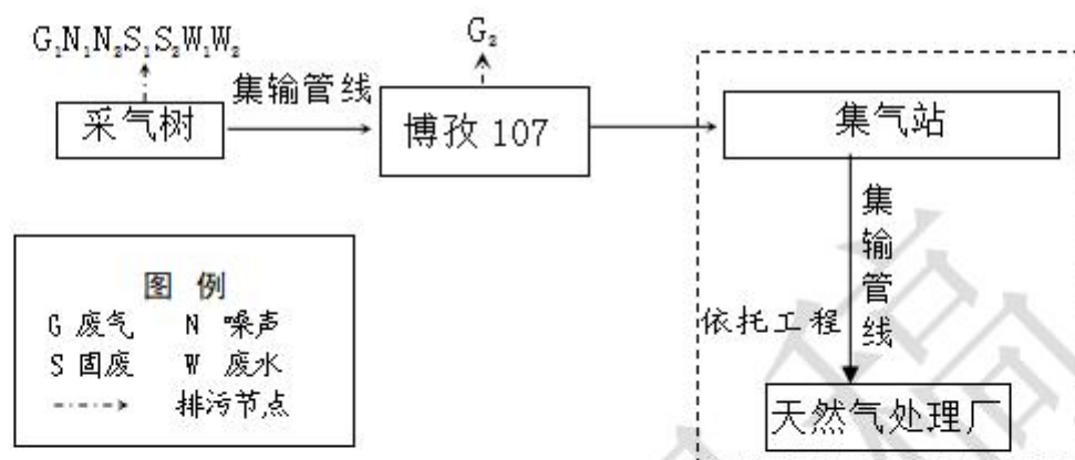
图 3.4-3 井场油气开采及集输工艺流程图
