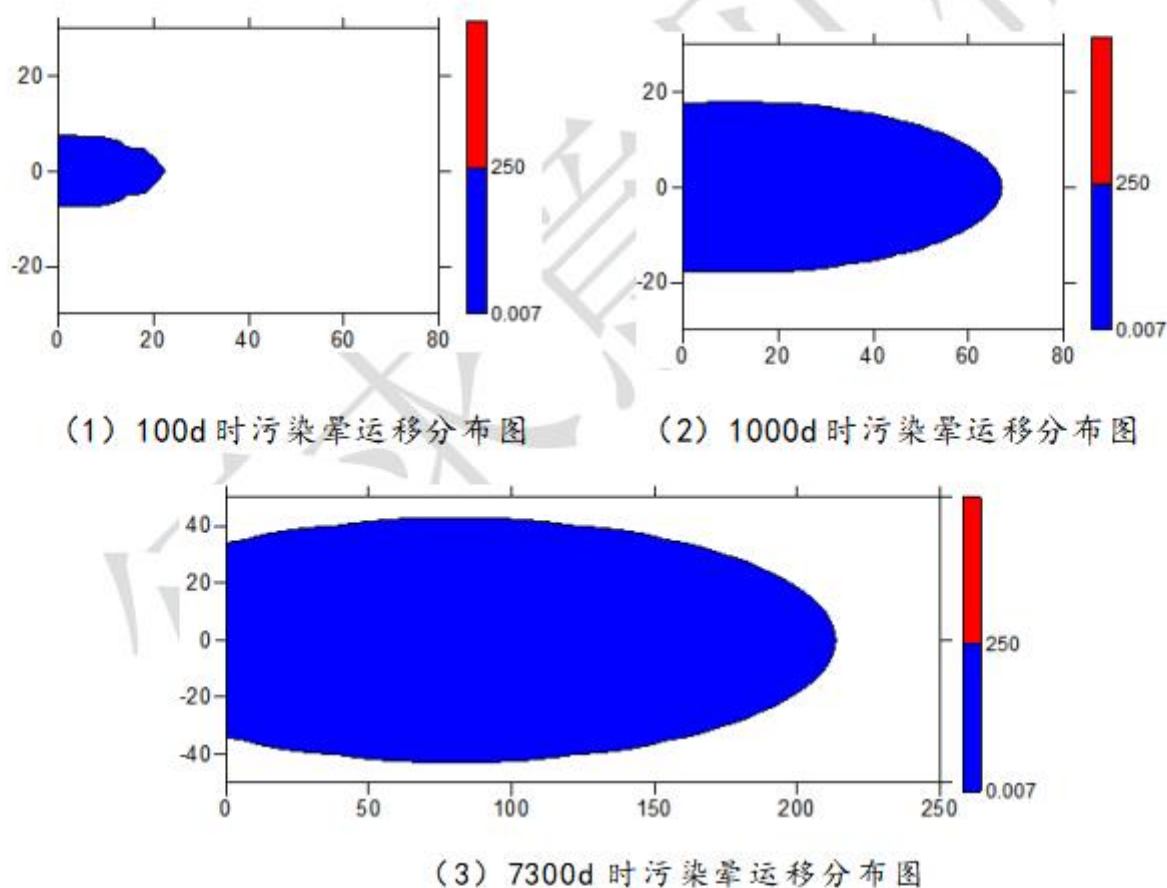
图 5.2-3 非正常状况下, 氯化物渗漏含水层影响范围图
