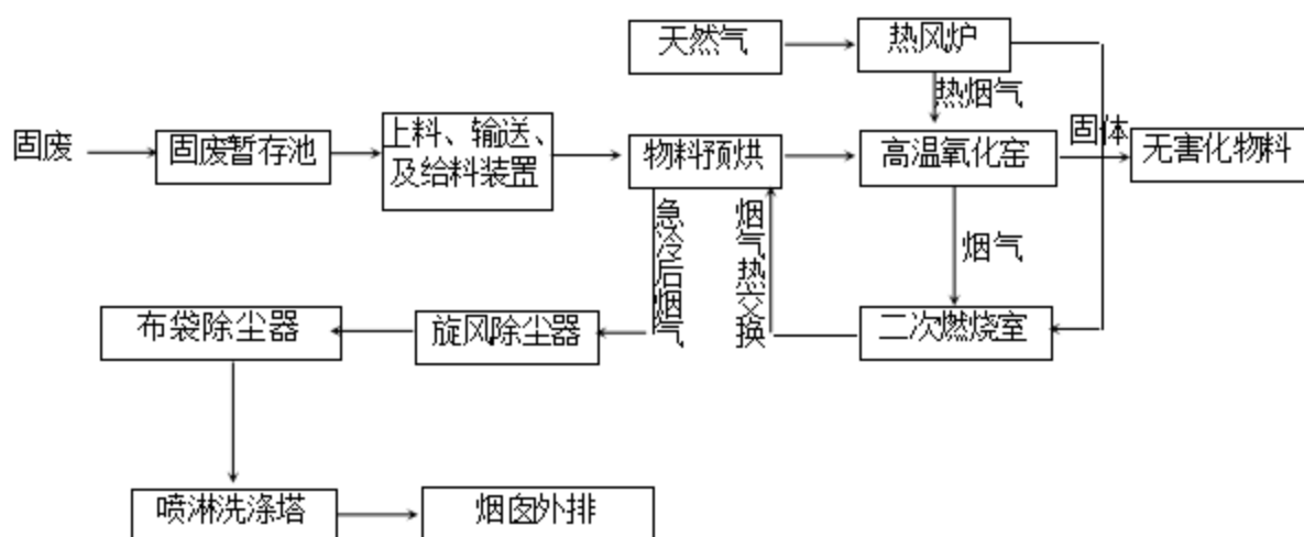
图 3.3-3 钻井聚磺体系岩屑固废处理工艺流程图
