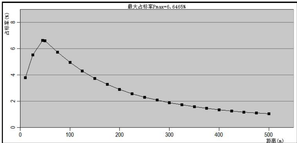
图 2.4-2 牙哈集中处理站无组织废气占标率-距离曲线图
