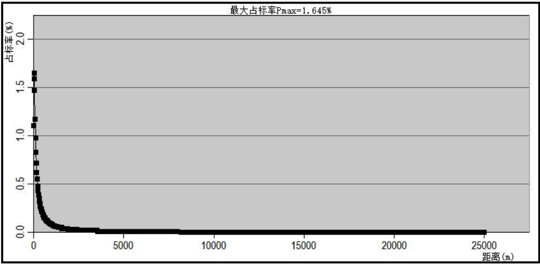
图 2.4-1 1#阀组无组织废气占标率-距离曲线图
