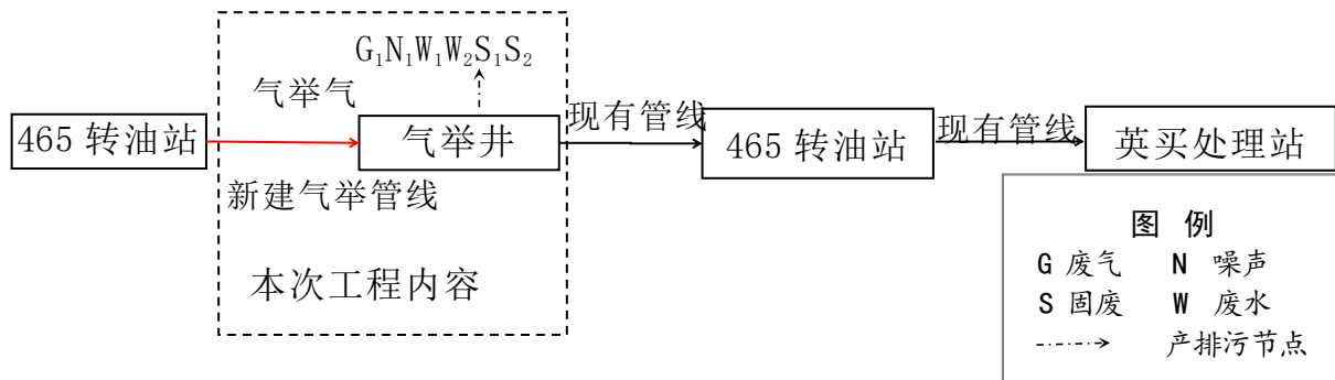
图 3.4-3 井场油气开采及集输工艺流程图
