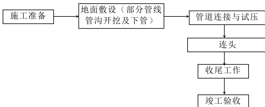
图 3.4-1 施工方案工艺流程图
