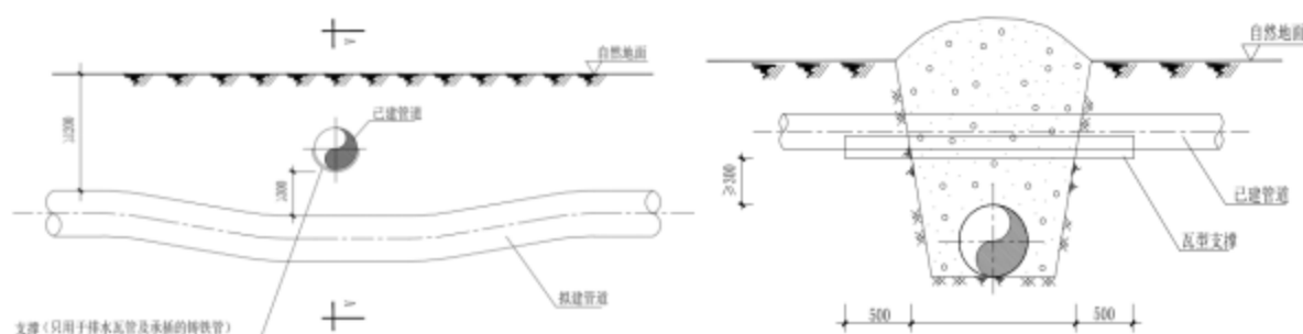
图 3.3-4 一般地段管道施工方式断面示意图
