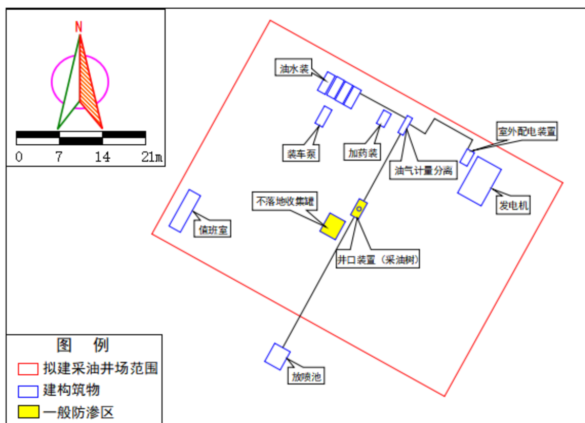
图 5.2-4 运营期井场分区防渗图
