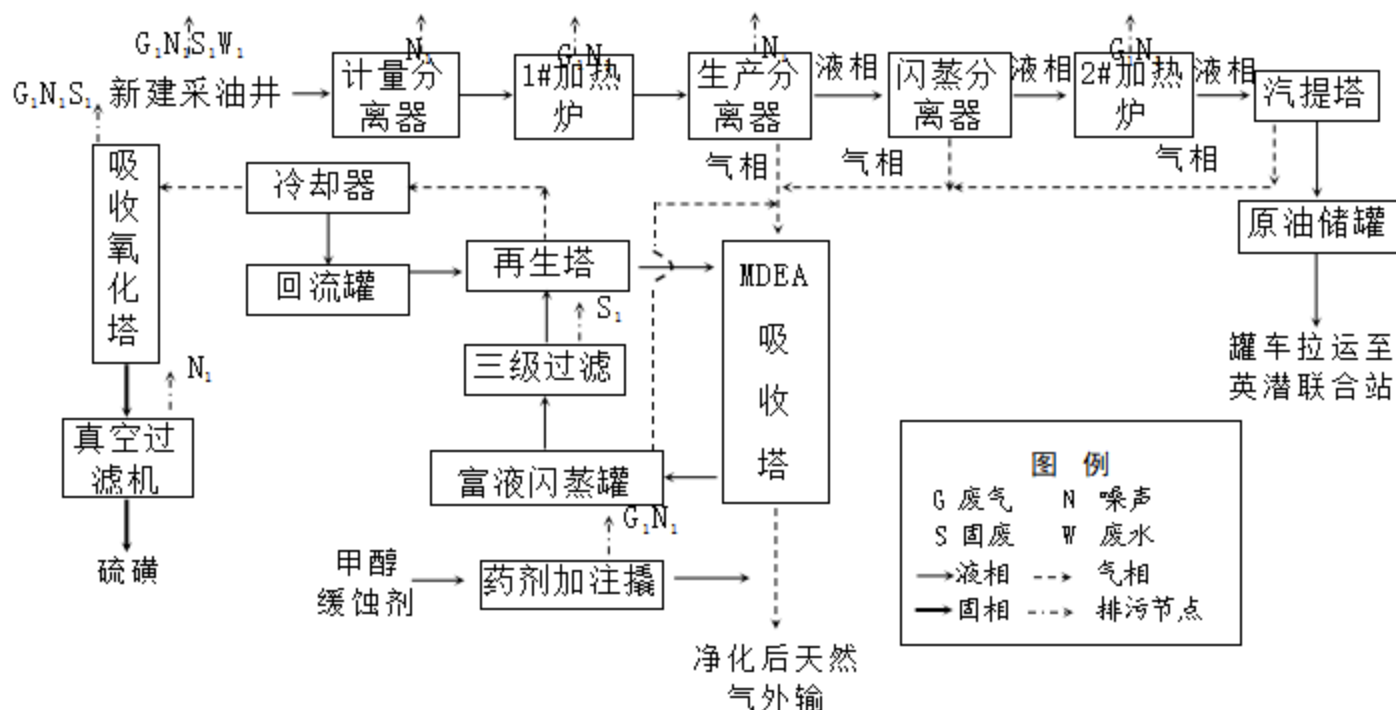
图 3.4-5 油气开采、处理及集输工艺流程图
