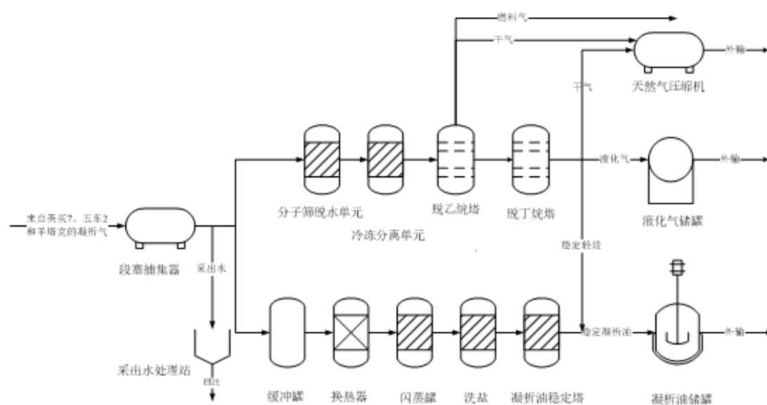
图 3.3-5 英买处理站油气处理流程图
