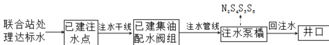
图 3.4-4 注水工艺流程图
