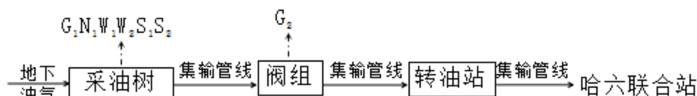
图 3.4-3 采油井场油气开采及集输工艺流程图
