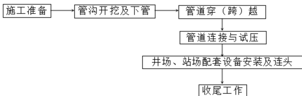
图 3.5-1 施工方案工艺流程图
