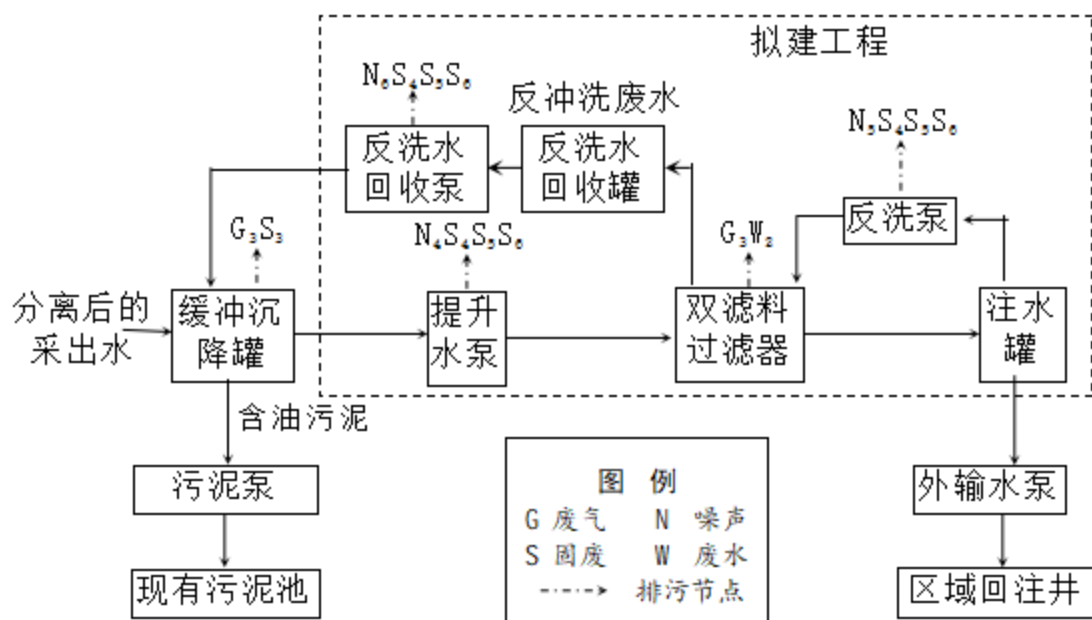
图 3.4-6 热普转油站采出水处理工艺流程图
