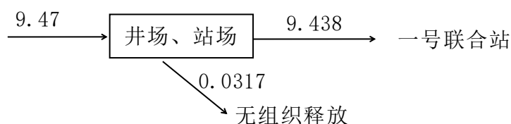
图 3.4-1 本项目硫平衡图 单位：t/a
