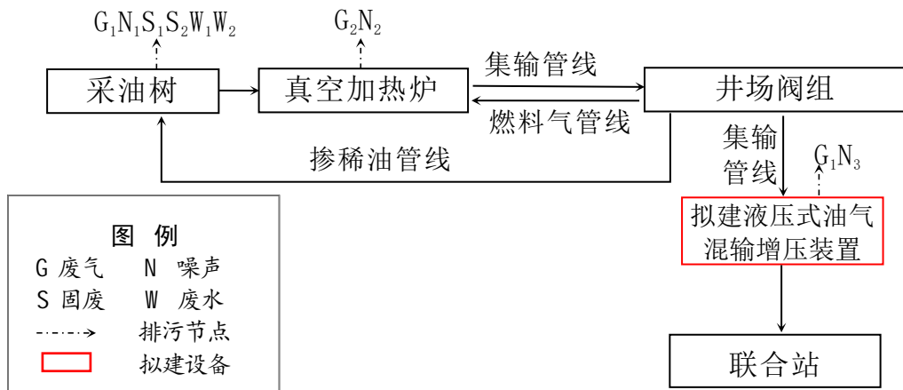
图 3.3-5 新建井场工艺流程图
