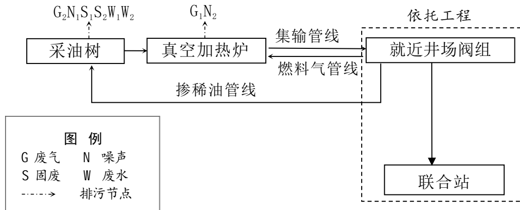
图 3.3-5 新建井场工艺流程图
