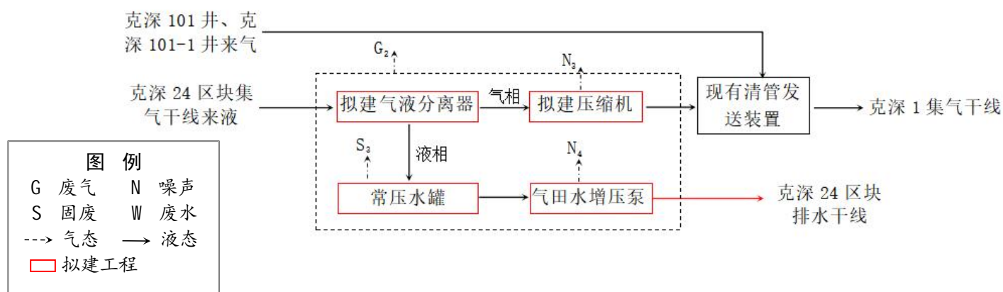
图 3.4-8 克深 1 集气站工艺流程图
