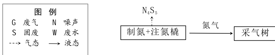
图 3.4-7 注气井场工艺流程图
