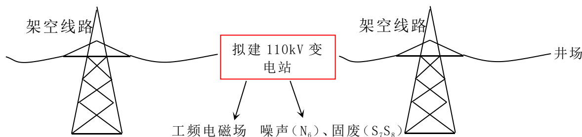
图 3.4-10 本项目变电站工艺流程与排污环节图
