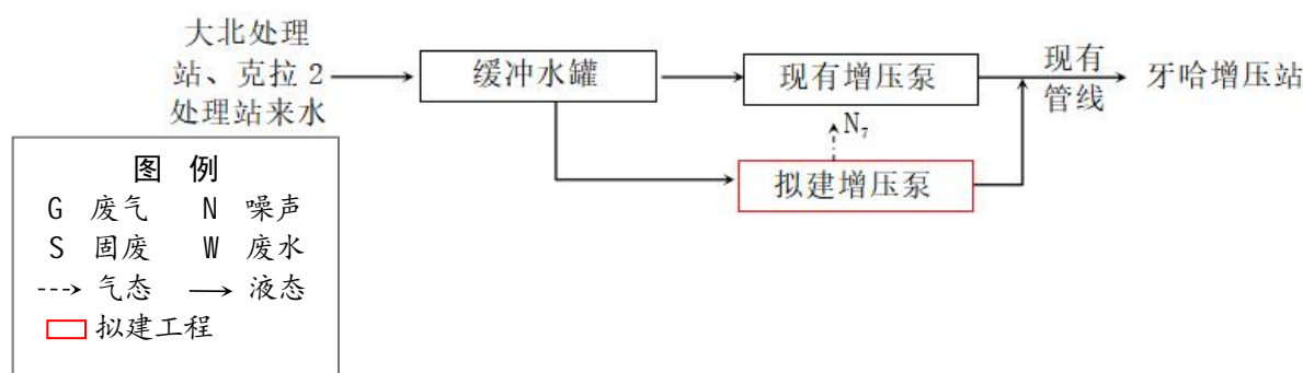
图 3.4-9 克拉增压站工艺流程图
