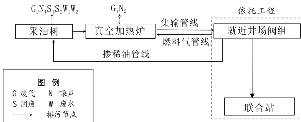
图 3.3-5 新建井场工艺流程图
