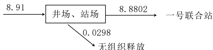
图 3.4-1 本项目硫平衡图 单位：t/a
