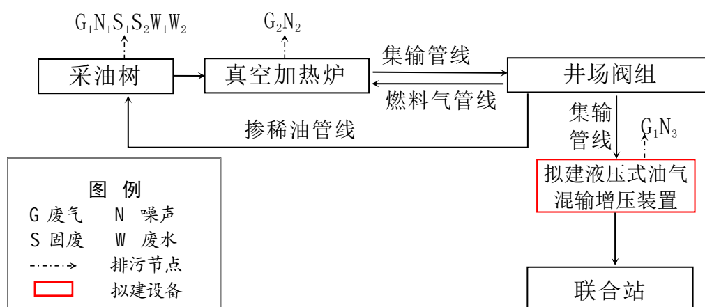
图 3.3-5 新建井场工艺流程图
