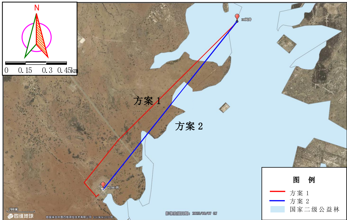
图 2.7-1 线路比选方案示意图
